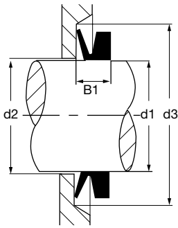
Fig. 17 Indbygningsdimension
