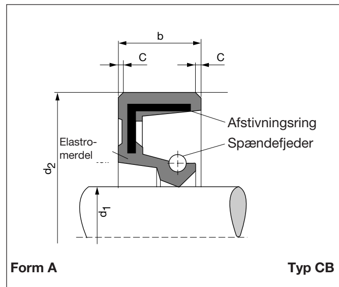
Fig. 1: Tætningsring uden beskyttelseslæbe
