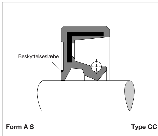
Fig. 2: Tætningsring med beskyttelseslæbe. Øvrige mål og oplysninger som form A
