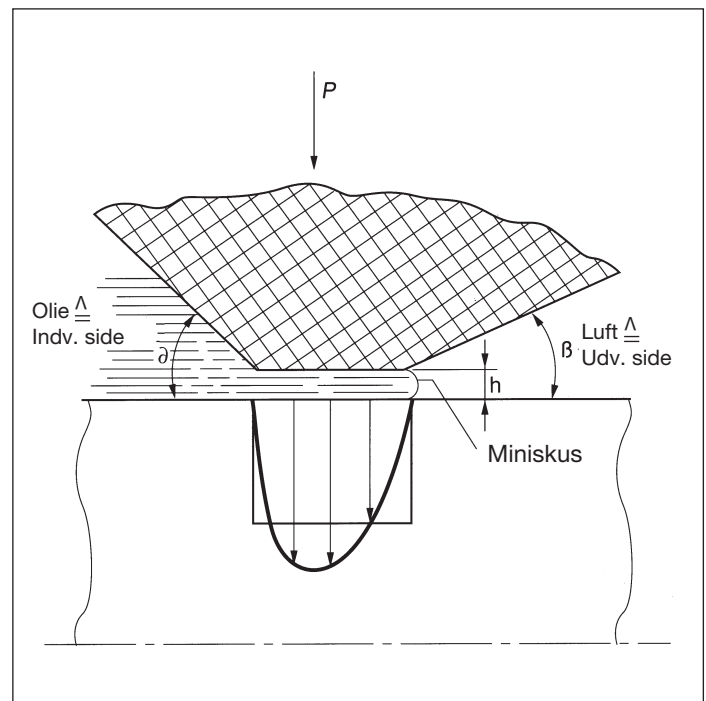
Fig. 1 Trykfordeling under tætningskanten
